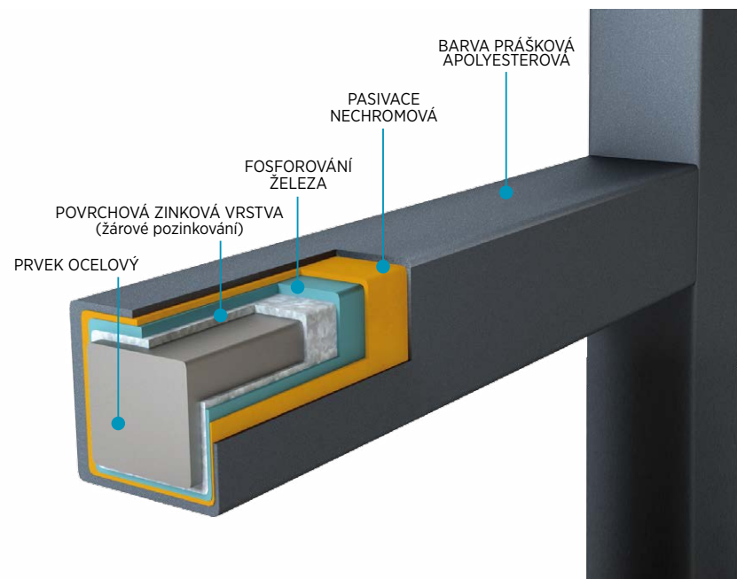
Průřez prvkem zabezpečený v systému DUPLEX
